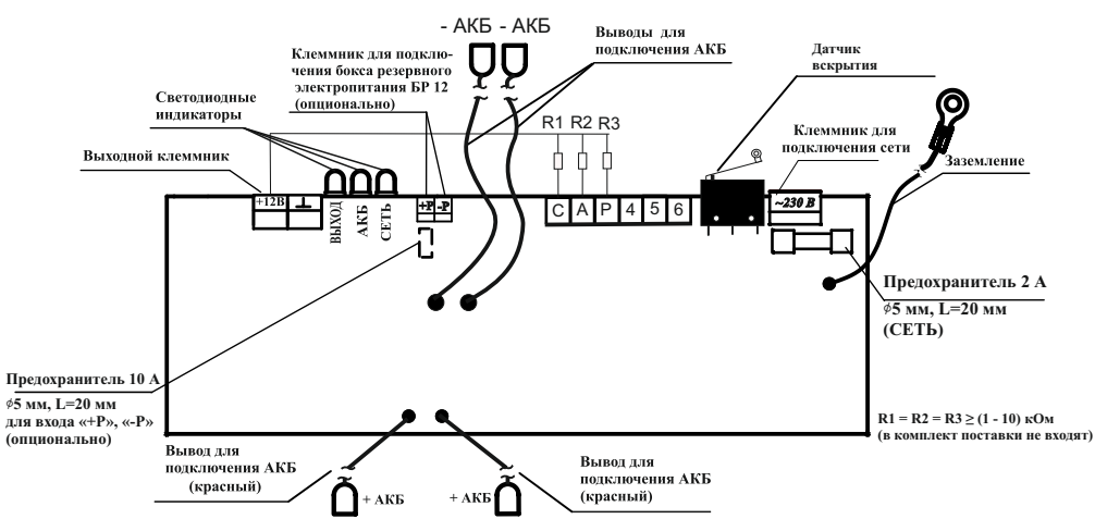
Рисунок 1 - Плата источника
